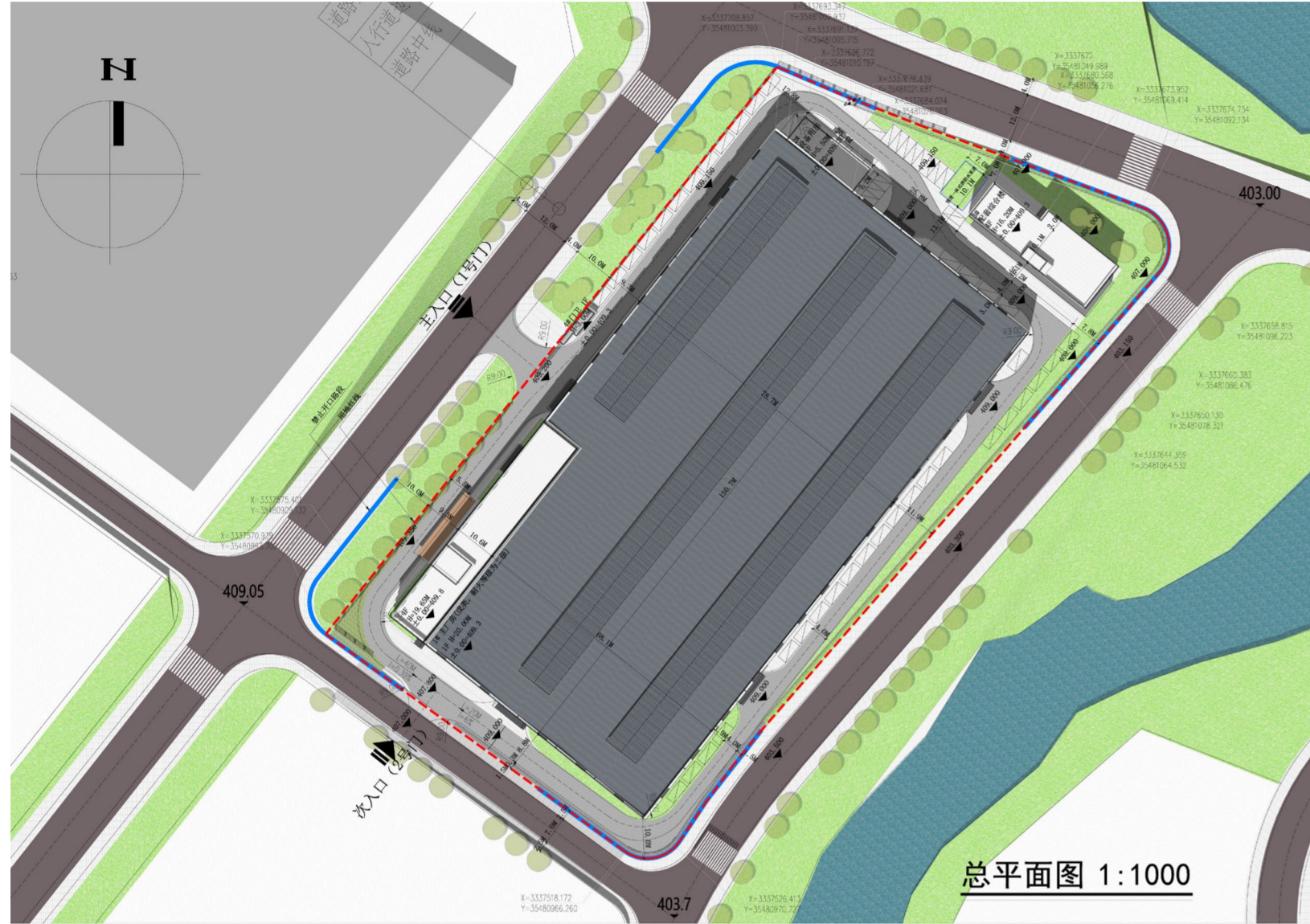
建筑工程规划总平面图
